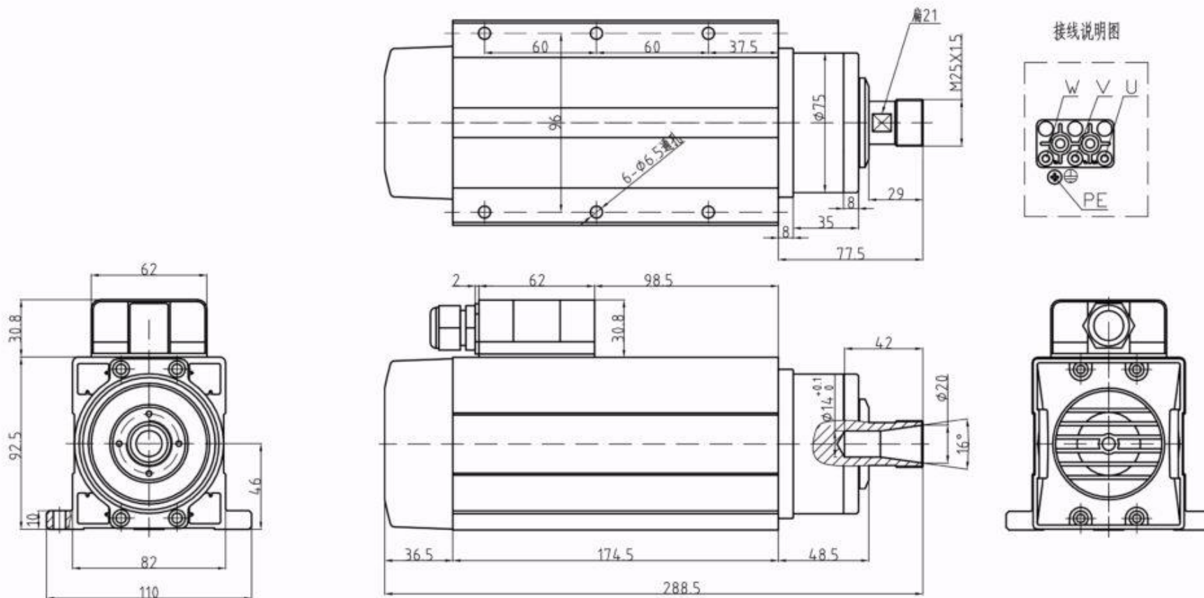
GDF46-18Z/2.2 220V接线盒外形图
