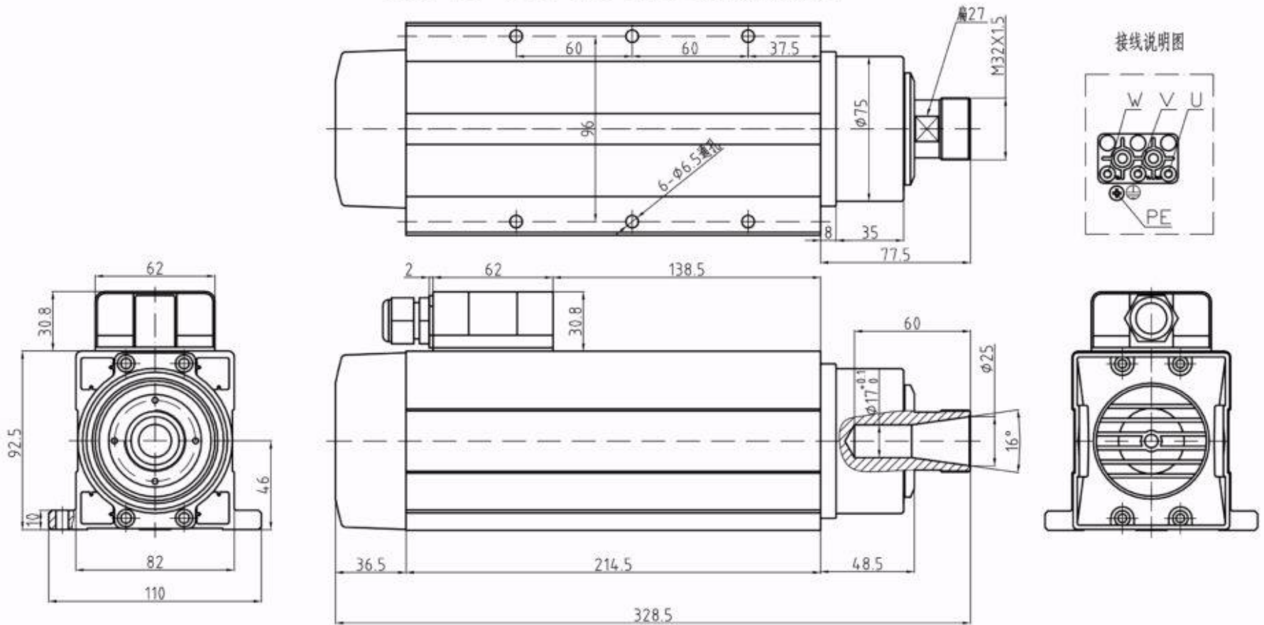
GDF46-18Z/3.5 380V接线盒外形图
